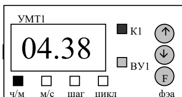
Рис. 2а. Лицевая панель прибора УМТ1.
